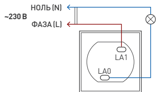
Рис. 1. Схема подключения одноклавишного выключателя
