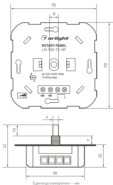
Едицица измерения — мм Рисунок 1. Габаритные размеры панели LN-500-TE-NF.
