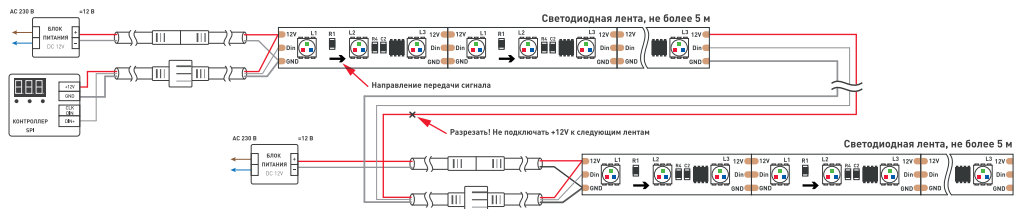
Рис. 1. Схема подключения ленты SPI-PFS-B60 с использованием SPI-контроллера с одним выходным портом и с использованием отдельных блоков питания
