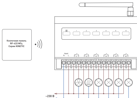
Рисунок 1. Пример схемы подключения релейного модуля TY-706-WF-SUF.
