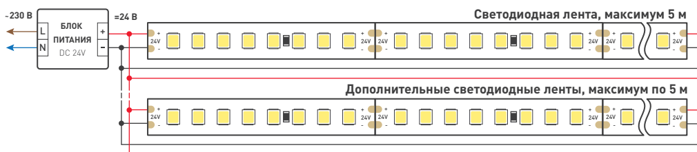
Схема 1. Подключение нескольких светодиодных лент с двух сторон для обеспечения равномерного свечения ленты по всей длине.
